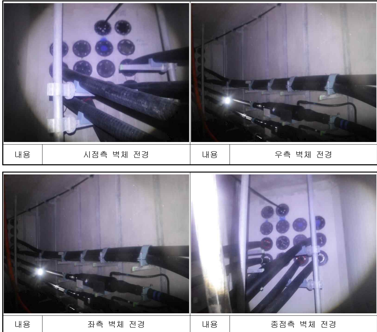
[사진 4.29] 남면~백석#6 전경
