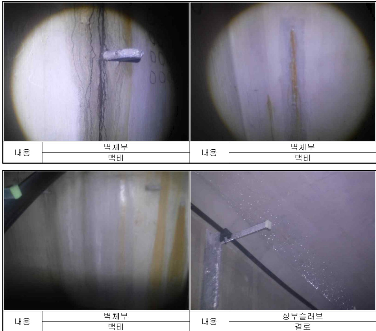
【사진 4.62】 맨홀 내부 주요 손상
