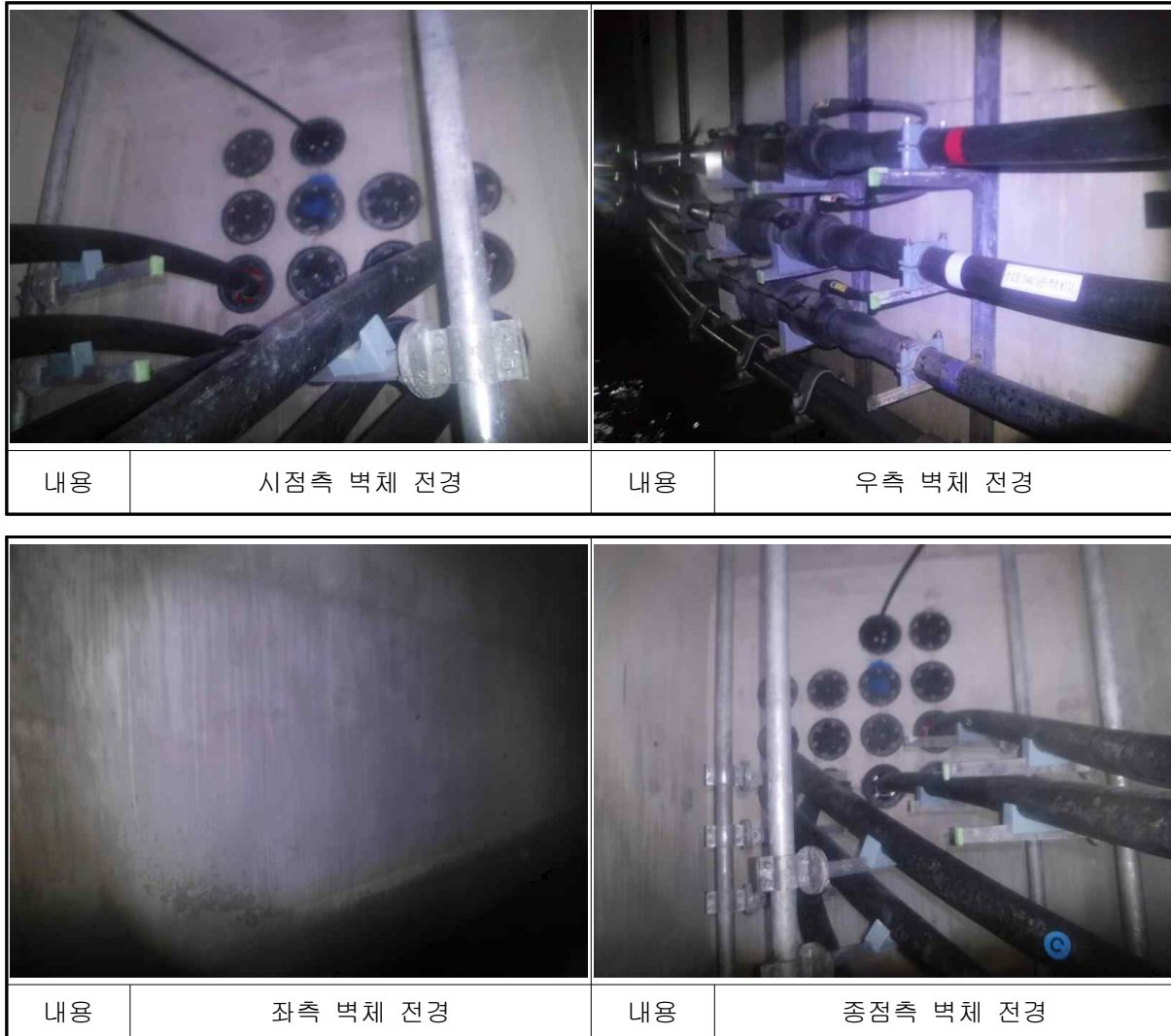
[사진 4.37] 남면~백석#8 전경
