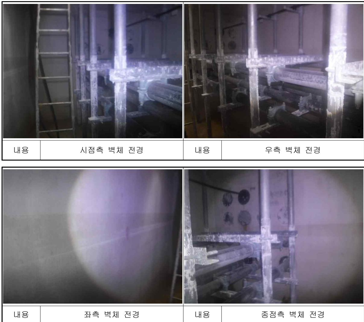
[사진 4.89] 남면~백석 활락#5 전경
