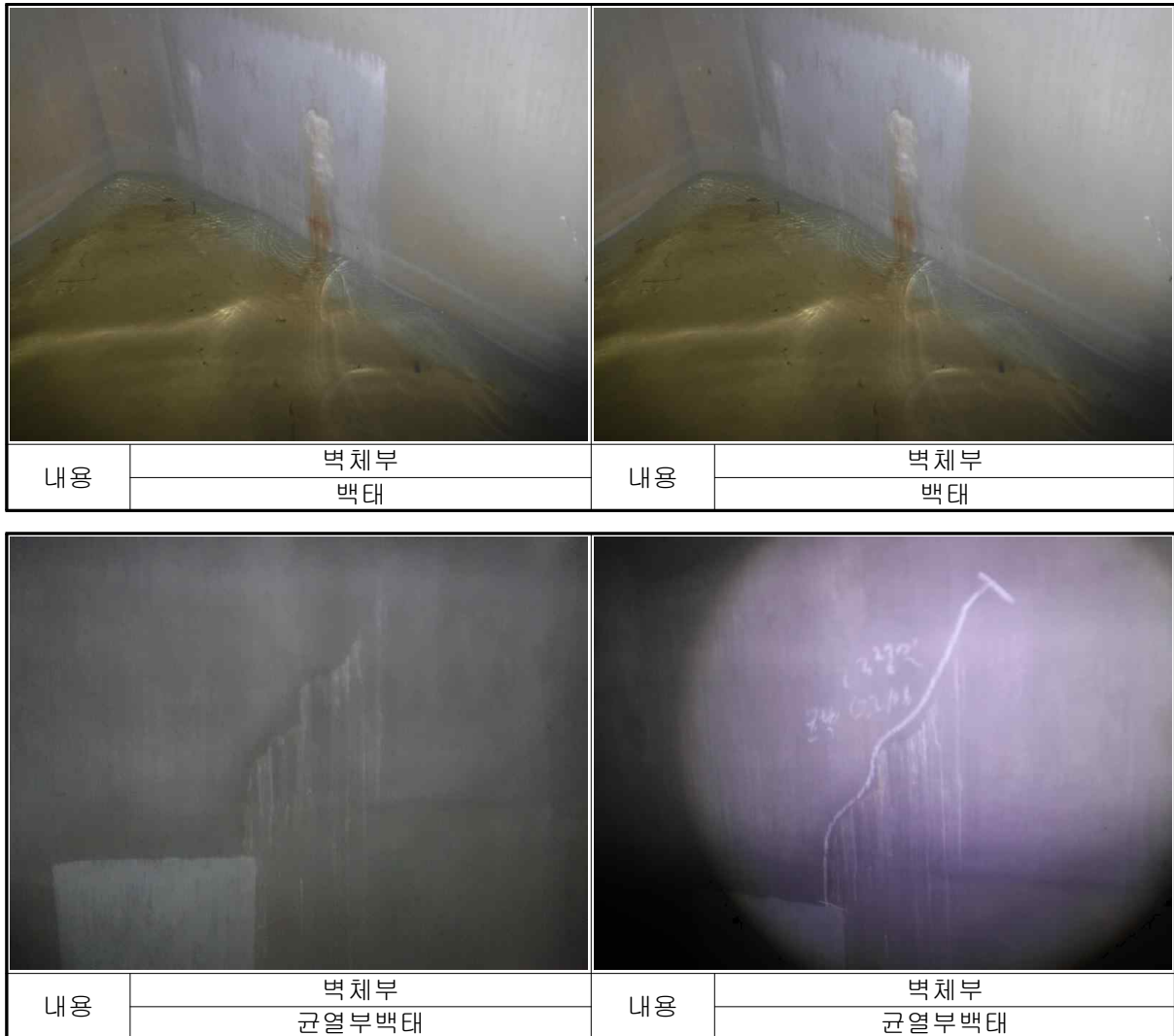
【사진 4.22】 맨홀 내부 주요 손상
